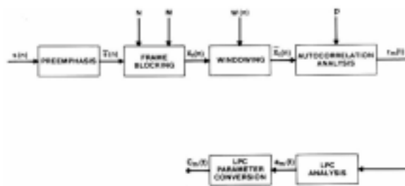
Gambar 3. Blok Diagram Prosesor LPC
