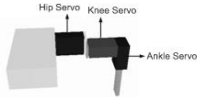
Gambar 3. Bagian-bagian pembentuk kaki robot
