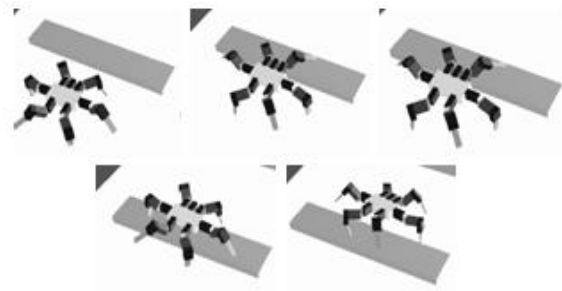
Gambar 17. Simulasi robot melewati halangan rendah setinggi 5 cm
